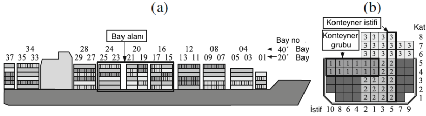
Şekil 4: Bir Geminin Depolama Yapısı (a) ve Yuvarının En Kesit Görünüşü (b).
